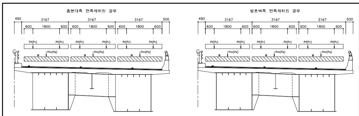
〈그림 6.7〉 설계활하중 재하의 경우
