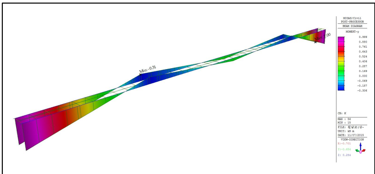
<그림 6.12> 단위모멘트 하중에 의한 모멘트도(영향계수 K )
