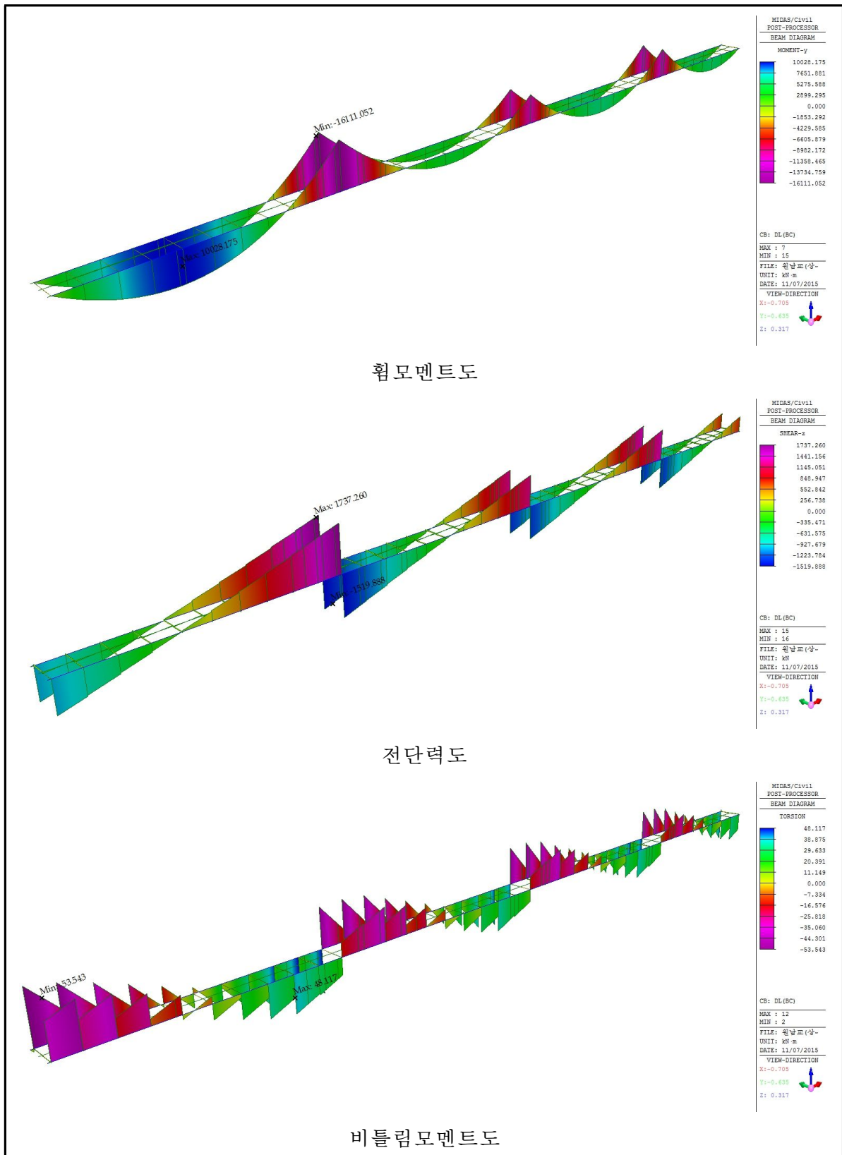
〈그림 6.9〉 합성전 고정하중에 의한 단면력도
