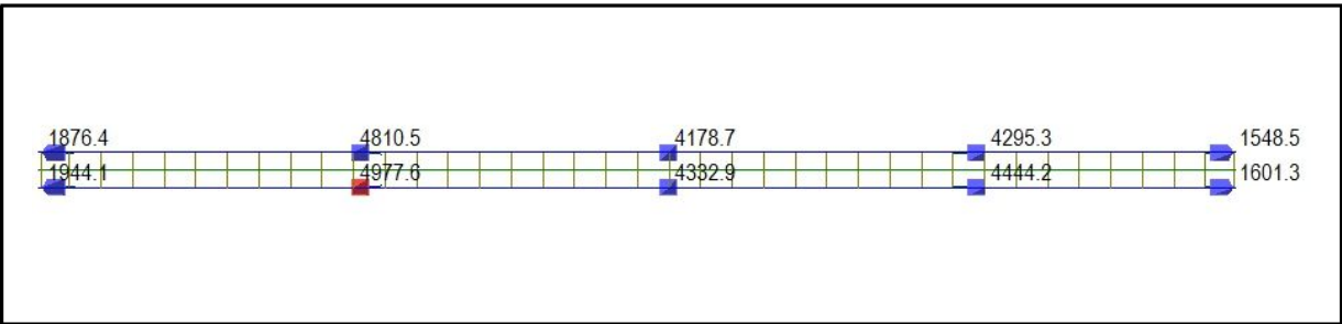
<그림 6.15> 고정하중+활하중에 의한 반력
