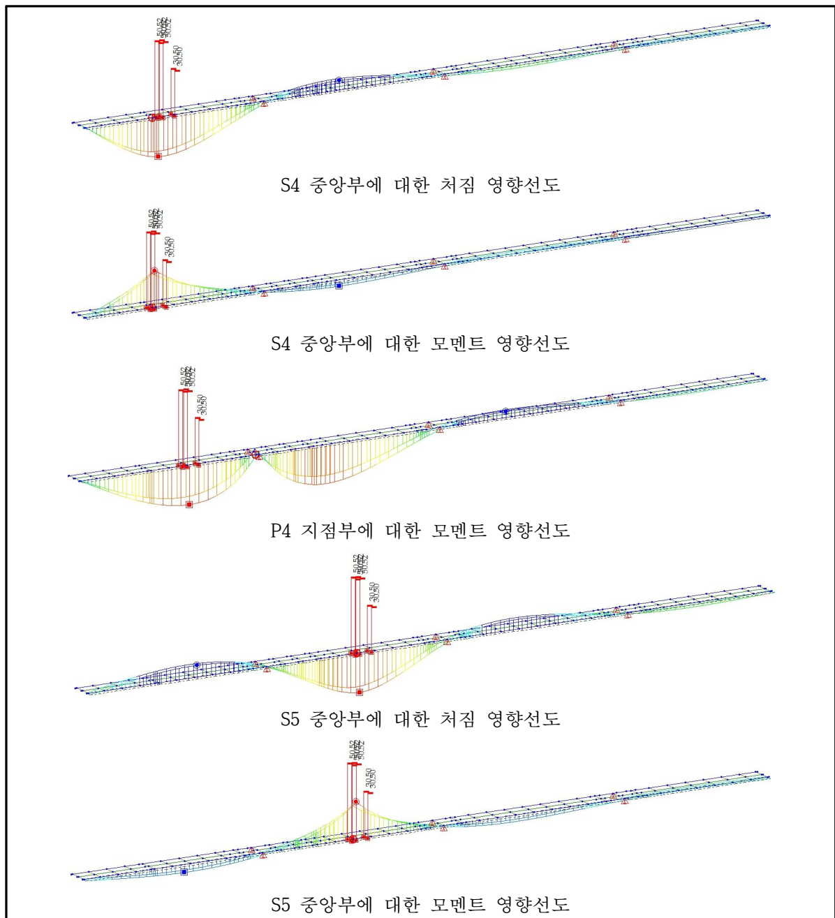
<그림 6.16> 위치별 영향선도
