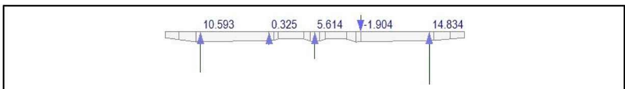
〈그림 6.6〉 합성후 고정하중에 의한 복부판의 반력
