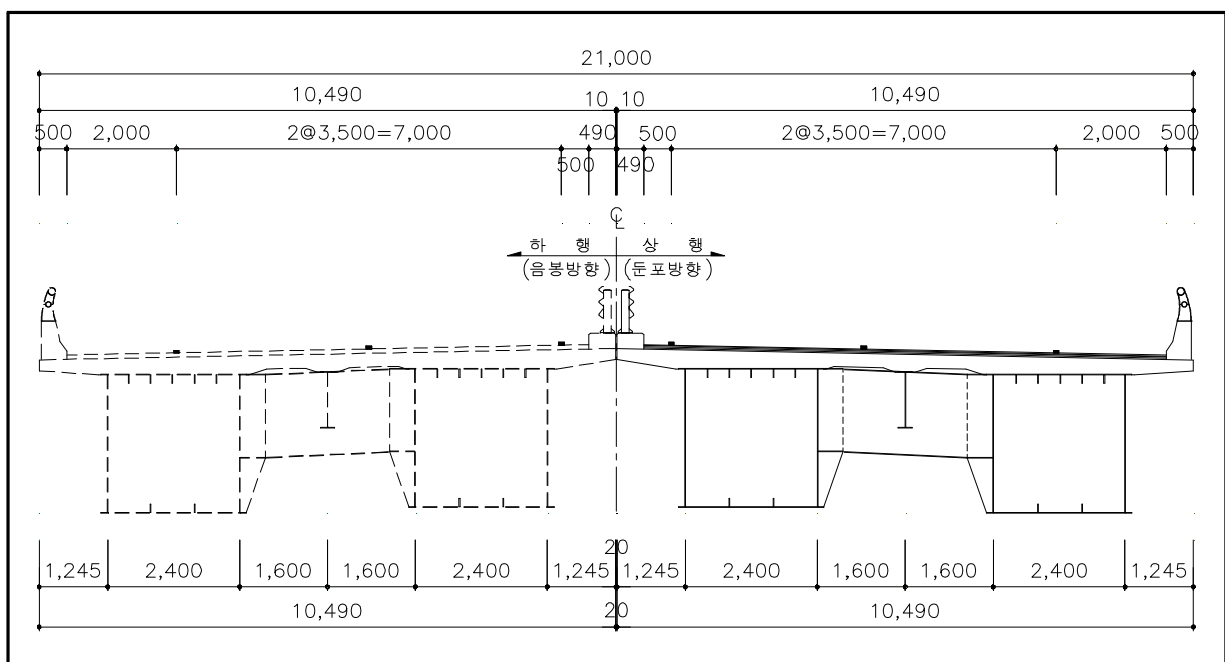
〈그림 6.3〉 구조해석 모델 횡단면도
