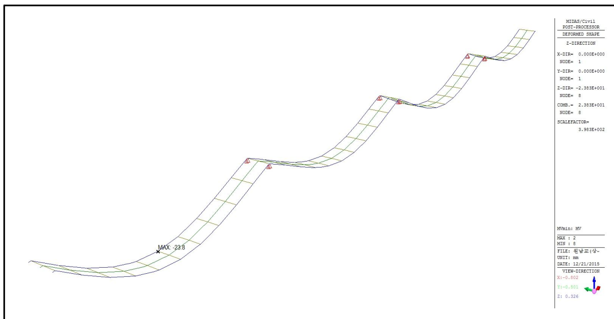
&lt;그림 6.13&gt; 활하중에 의한 주거더 처짐도 (충격포함)
