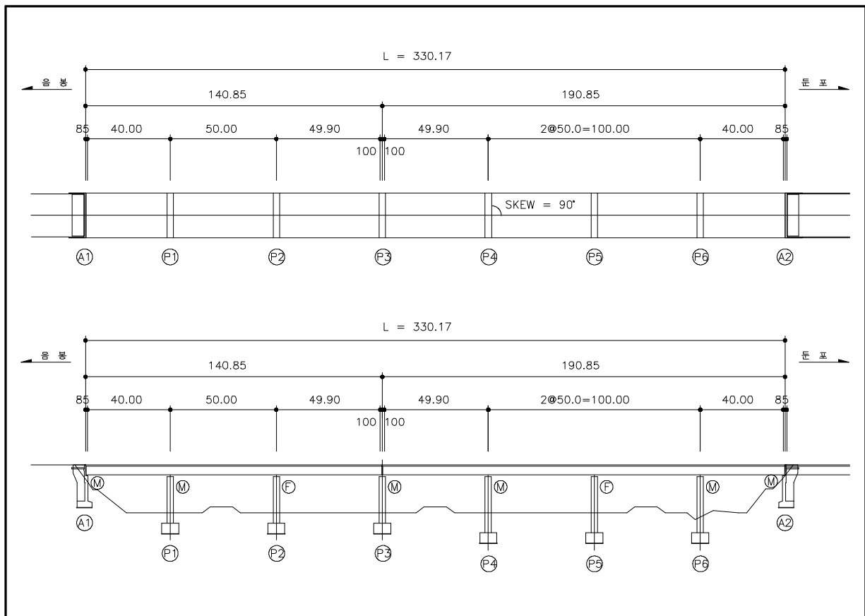
<그림 6.1> 원남교(상) 종평면도
