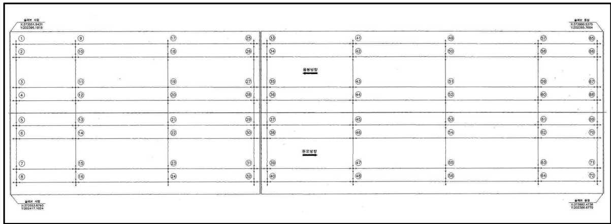
<그림 6.14> 받침배치도
