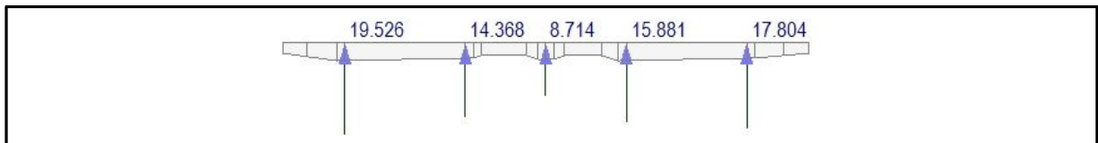
〈그림 6.5〉 바닥판 하중에 의한 복부판의 반력
